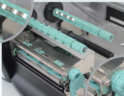
碳帶內外卷自動切換設計 安裝方便、使用簡單
